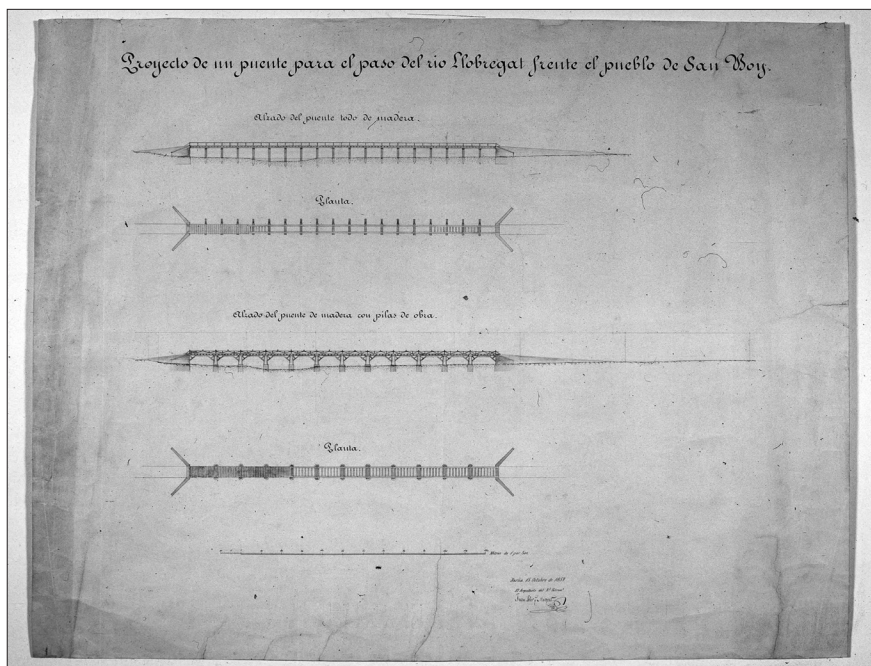
Fig. 5. "Proyecto de un puente para el paso del riu Llobregat frente al pueblo de San Boy" (1859) de l'arquitecte Juan Soler y Mestres. ACA, REAL PATRIMONIO, BGRP, Planos, 11 (1-2)
