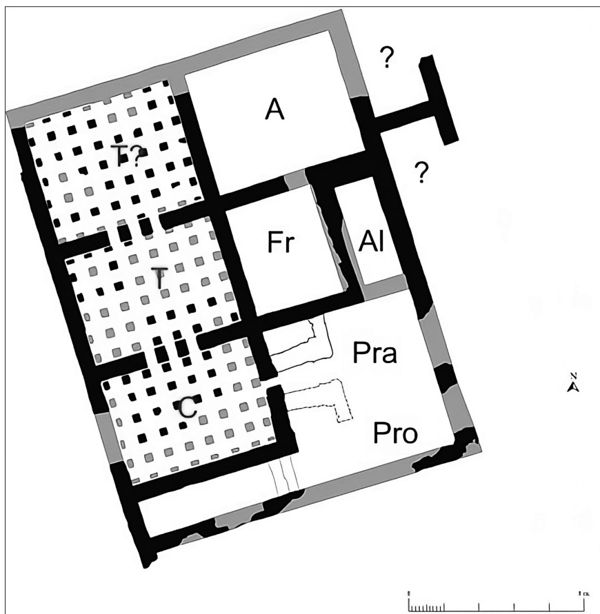
Figura 3. Vista en planta del balneum del segle I. (planimetria: E. Revilla, I. Camps i F. Boullosa)
