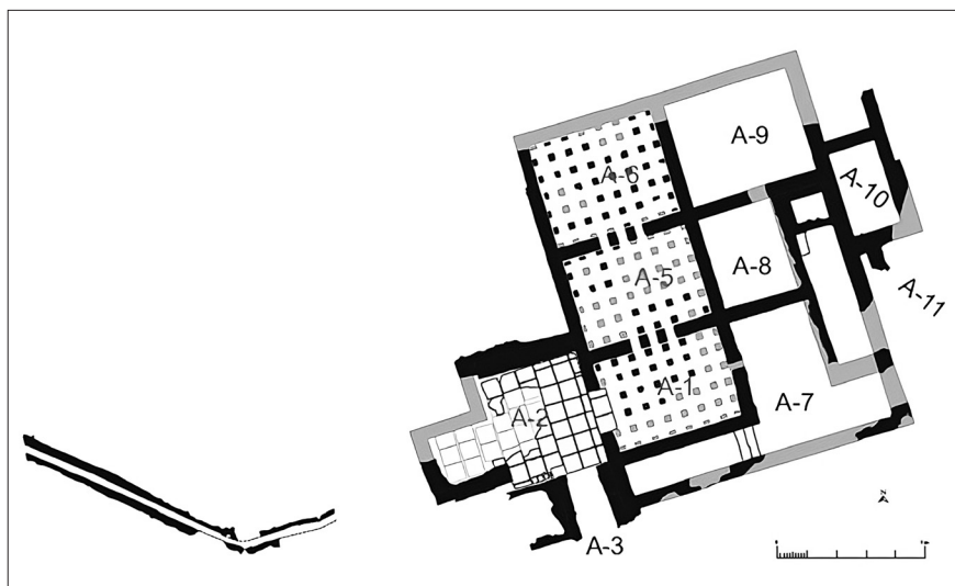
Figura 2. Vista en planta dels diferents àmbits documentats, a l'esquerra es pot veure la claveguera associada a les termes (planimetria: E. Revilla, I. Camps i F. Boullosa)*.
